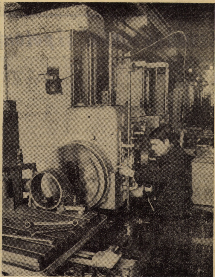
Printr-o amplasare judicioasă a utilajelor de bază și folosirea rațională a spațiilor de producție, la I.U.P.S. Sibiu fluxul tehnologic a cunoscut o îmbunătățire substanțială Foto: FRED NUSS
