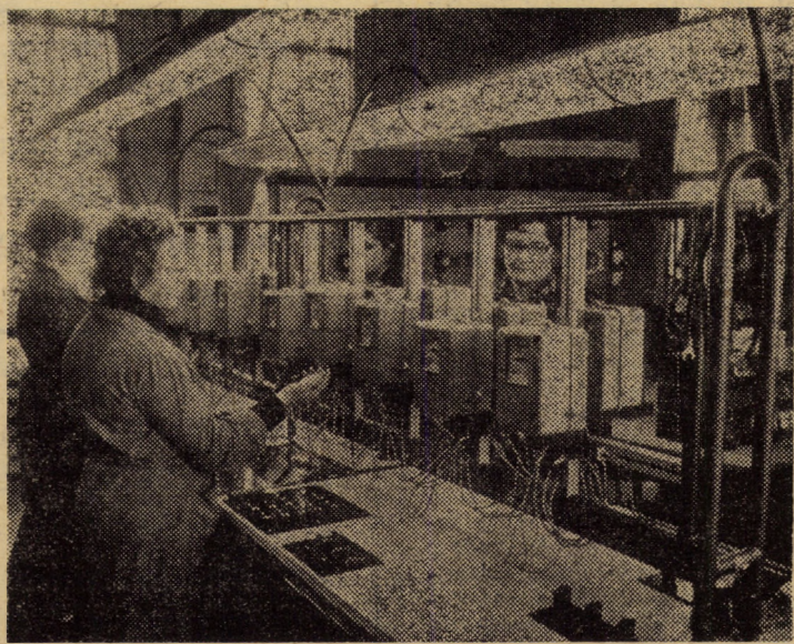
Verificarea metrologică a contoarelor trifazice în sala de etalonare și verificare aparate de măsură de la I.R.E. Sibiu
