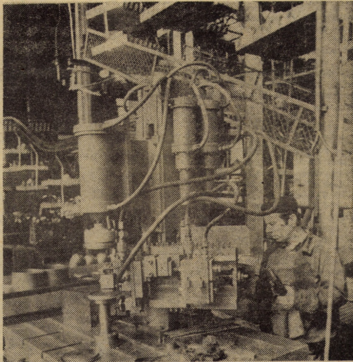
Printre utilajele realizate prin autoutilare la întreprinderea „Email roșu” Mediaș figurează și dispozitivul de tăiat-bordurat vase emailate cu acțiune simultană, realizîndu-se importante economii la muncă. Foto: FRED NUSS
