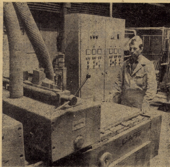
Unul din utilajele de mare productivitate ale sectorului finisaj de la I.P.L. Sibiu — Fabrica de mobilă Mediaș: Mașina de lustruit cu 6 cilindri, la care se execută lucrări de finisaj cu lacuri poliesterice.
