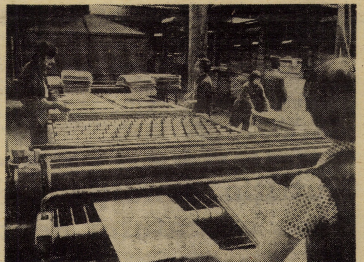
Întreprinderea I.P.L. Sibiu, Fabrica de mobilă Mediaș, sectorul finisaj. Aplicarea mecanizată a adezivului pe panourile ce urmează a fi furnizate pe ambele părți — fază pregătitoare pentru presa termică monoetajată cu timpi scurți de presare. Foto: Fred NUSS
