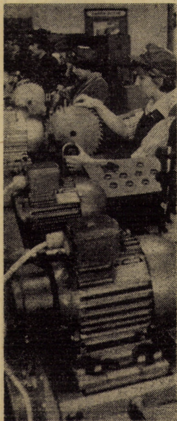
Mașini moderne de ascuțit fețe laterale la plăcuțe din carburi metalice - utilaje realizate la I.U.P.S. Sibiu Foto: FR. NUSS
