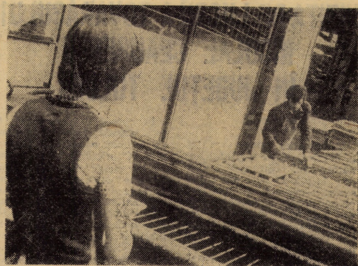
La I.P.L. Sibiu, Fabrica de mobilă Mediaș, operațiunile de finisaj sint executate în bună parte mecanizat. În fotografie: aplicarea adezivului pe panourile ce urmează a fi furnizate pe ambele părți, pregătite pentru presa termică monoetajată. Foto: FRED NUSS
