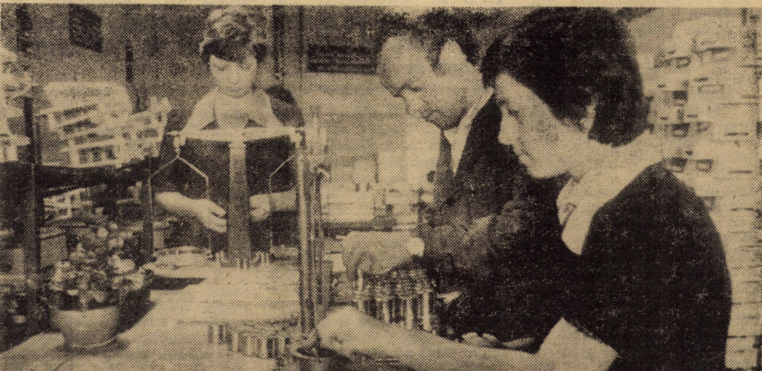
Întreprinderea „Balanța” Sibiu. Linia de montaj balanțe pentru gospodărie (uz casnic) al cărei colectiv de muncitori, în urma bunelor rezultate obținute, se înscrie printre cele fruntașe din cadrul secției a II-a.
