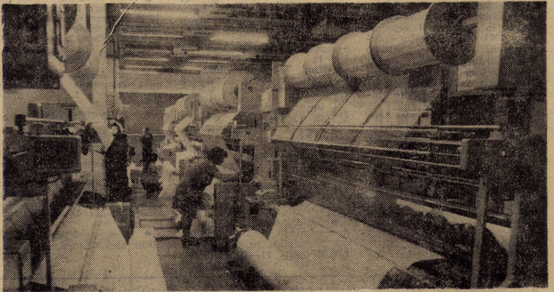
Noile utilaje de mare randament — mașini de tricatat rapide cu urzeală — instalate în decursul trimestrului III a.c., la întreprinderea „Drapelul roșu”, unitatea I, din Sibiu, prezintă posibilități multiple de realizare a unor tricaturi de o mare diversitate. Foto: FRED NUSS
