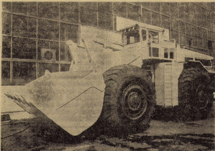
Încărcător frontal de 16 m.c.
