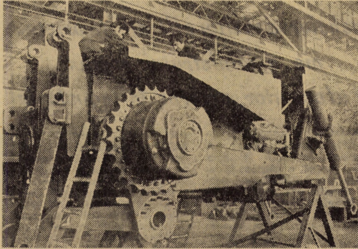
Buldozer pe șenile cu motor de 550 CP aflat în aceste zile în ultimele faze de montaj
