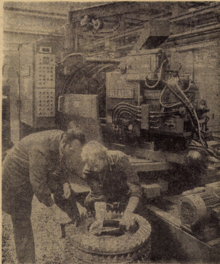
În secția de prelucrări mecanice a Întreprinderii mecanice Mirșă, utilaje moderne și de înaltă productivitate asigură prelucrarea co-roanei dințate de la punțile motoare ale autobasculantelor grele. Foto: FRED NUSS
