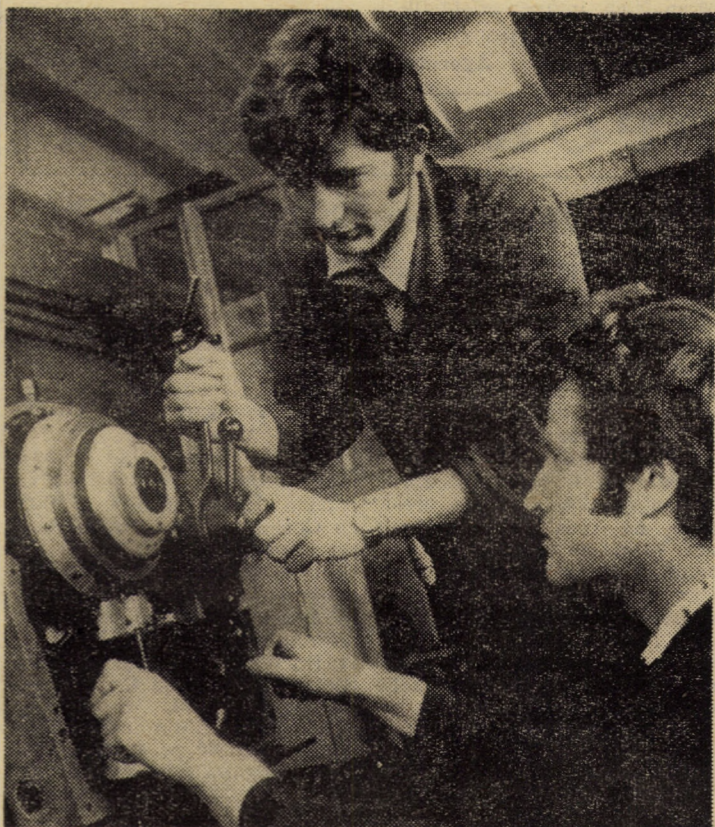
Reglarea și verificarea, la standul de probă, a instalației hidraulice pentru mașinile de rectificat universale, efectuată de lăcătușii Stelian Popa și Iacob Ghișoiu din secția hidropneumatică a întreprinderii „Balanta” Sibiu
