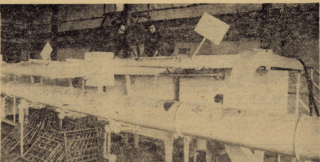
În prezent, la întreprinderea „Balanța II“ Sibiu se află în probe tehnologice o instalație de curățire chimică a pieselor turnate, realizată prin autototare. Cu ajutorul noului utilaj, se îndepărtează, pe baze chimice, resturile de nisip, rezultate din turnare, proces care are loc fără consum de energie electrică
