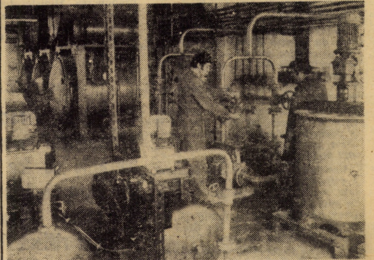
Prin darea în funcțiune a instalației pentru impregnat scindurele — aflată în prezent în probe tehnologice — din secția tratare și ameliorare a lemnului de la Fabrica de creioane a I.P.L. Sibiu, calitatea produselor va fi mult îmbunătățită, asigurîndu-se totodată o creștere a producției de cca 30 la sută. Foto: FRED NUSS
