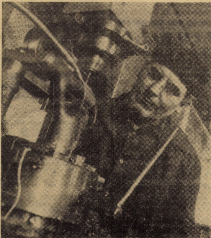
În cadrul atelierului prototipuri al sectorului unelte pneumatice de la întreprinderea „Independența” din Sibiu, muncitorul Ion Chețan execută lucrări de frezare la minerele ciocanelor cu acționare pneumatică. Foto: FRED NUSS
