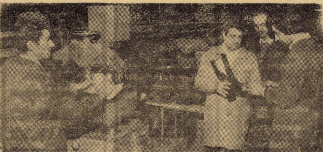
Schimbului condus de maestrul Gheorghe Schuster, de la F.I.P. Agnita, i-a revenit sarcina de a confecționa primele noi modele de cizme napa pentru producția internă a anului 1982. Pe linia tehnologică tras-tălpuit-finisaj, pe fiecare schimb, sînt confecționate peste 500 perechi cizme pentru femei
