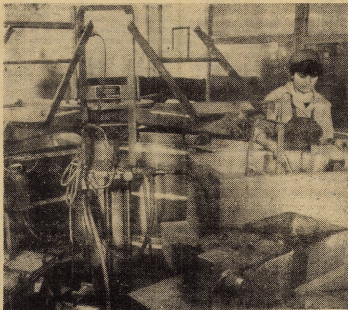
I.P.L. Sibiu, sectorul creioane. De curînd, la această unitate funcționează cu bune rezultate o instalație de degresat mine care spală într-un schimb cca 280 000 mine pentru creioane
