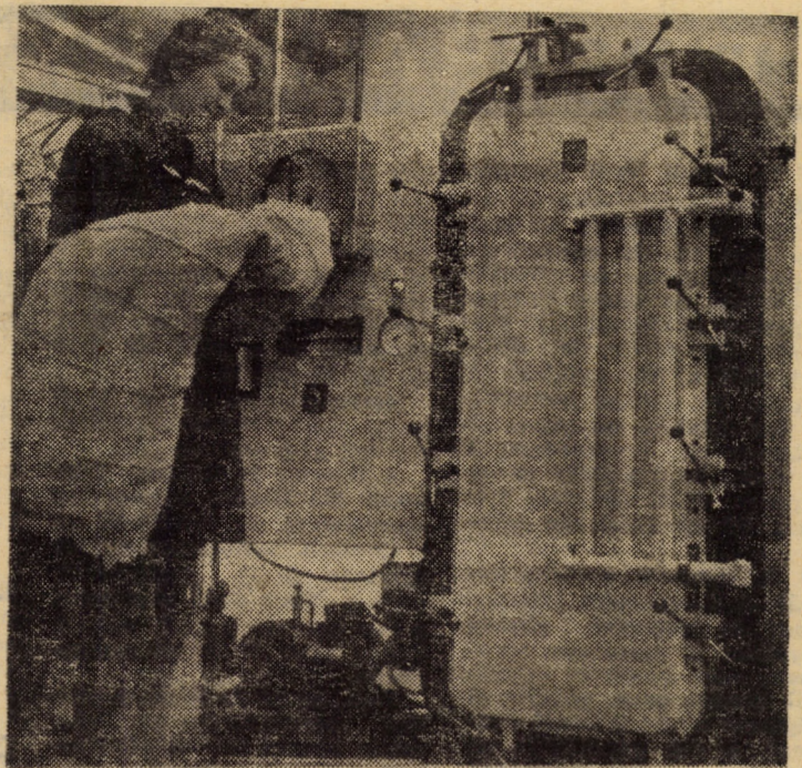
Întreprinderea „7 Noiembrie” Sibiu. Pentru a asigura ciorapilor din fire sintetice o bună stabilitate, aceștia sînt introduși, înaintea fazei confecționării, în autoclave speciale de prefixat unde are loc un proces de stabilizare Foto: FRED NUSS
