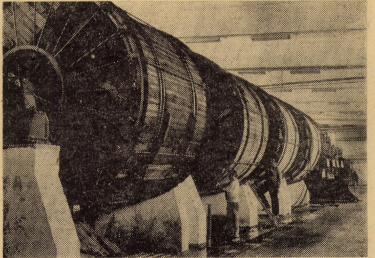
Întreprinderea „13 Decembrie” Sibiu, secția tăbăcării, un obiectiv industrial nou și modern Foto: FRED NUSS
