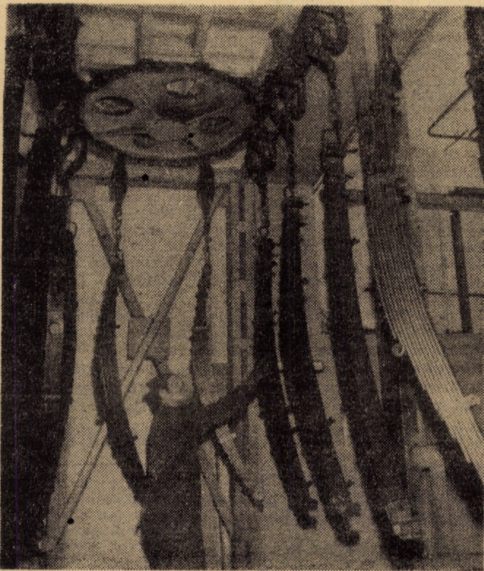
Recent, în secția arcuri lamelare de la I.P.A. Sibiu a fost dată în funcțiune o nouă linie de vopsit, amplasată pe 40 la sută din spațiul vechii vopsitorii
