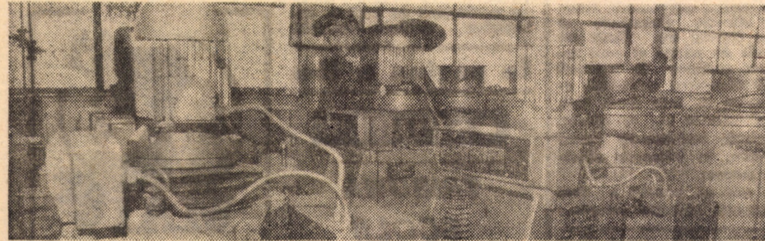
Mașini de rectificat capete de arcuri, realizate în scopul autoutilării la I.P.A. Sibiu
