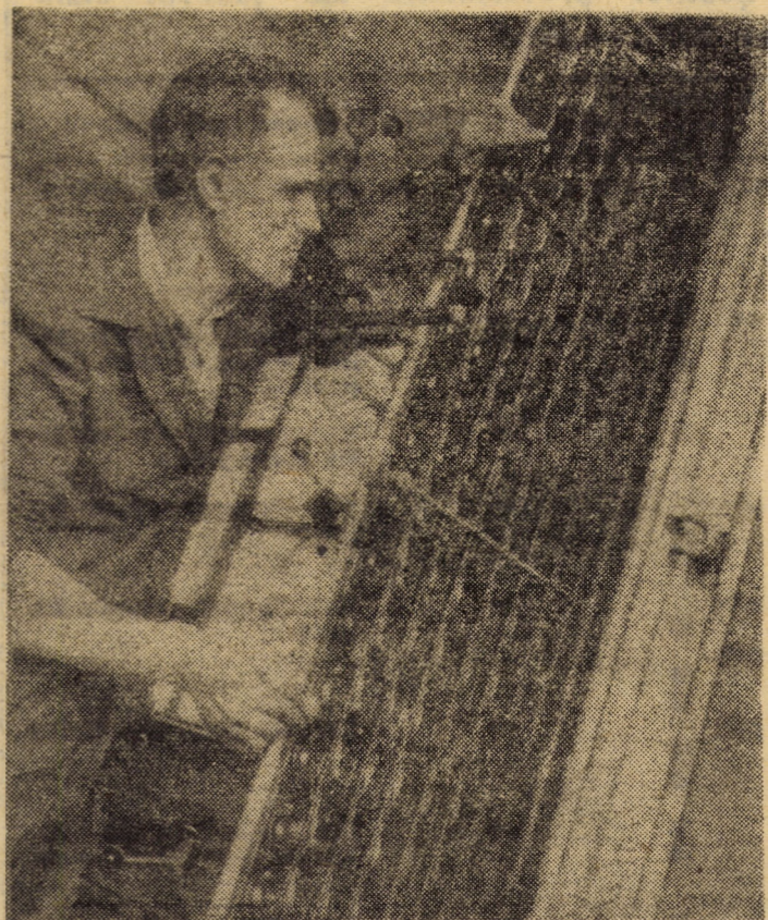
Recent, la întreprinderea „Libertatea” din Sibiu s-a realizat prin autoutilare o instalație de spălat băncile cu inele de la mașinile de răsucit și filat, folosindu-se ca agent de spălare apa și aburul, operație ce se efectua manual cu o cantitate însemnată de petrol Foto: FRED NUSS
