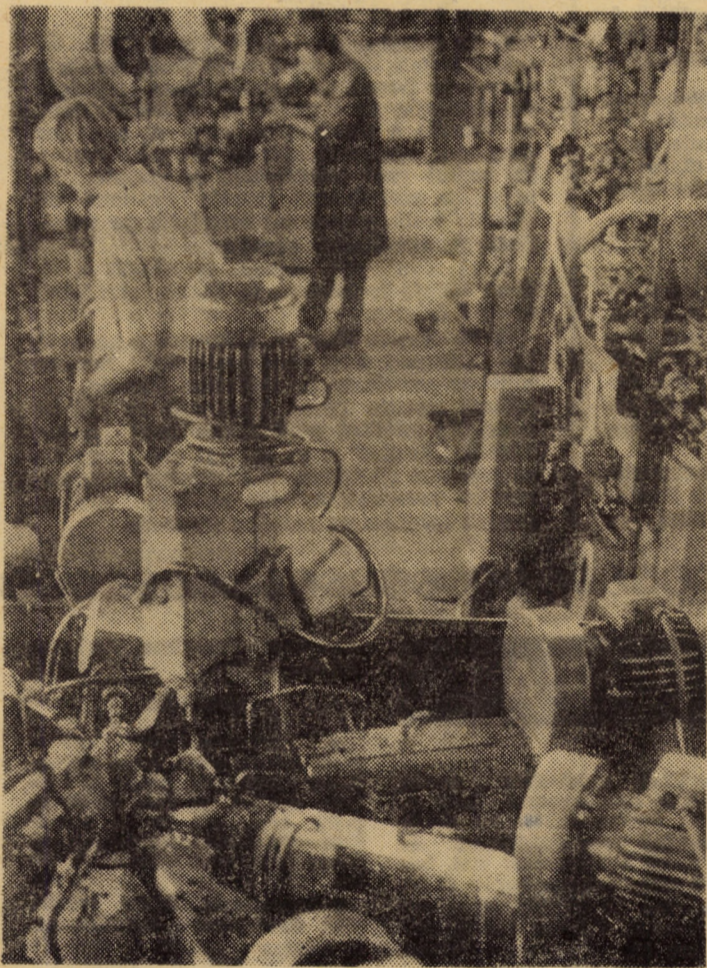
Prelucrări mecanice de înaltă precizie la întreprinderea de rele, Mediaș.
