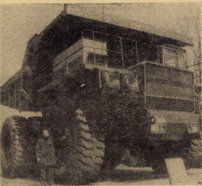
Un nou „mastodont” pe roți, produs de mare... greutate pentru economia națională: autobasculanta Diesel-electrică de 110 tone cu șasiu rigid
