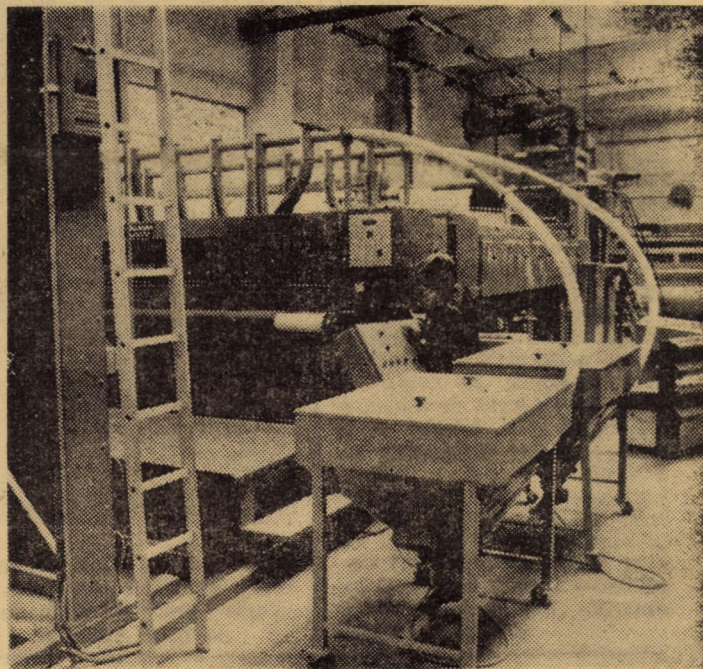
Recent, la întreprinderea textilă „Dumbrava” Sibiu a fost dată în funcțiune o mașină automată de finisat mochetă pentru autoturisme „OLCIT”. Noul utilaj depune un strat de polietilenă pentru fixarea texturii. Foto: FR. NUSS
