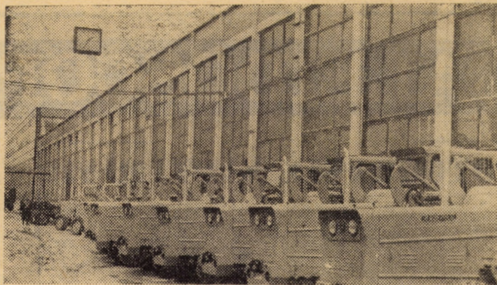
Unul dintre cele mai reprezentative produse ale colectivului de la I.U.P.S. Sibiu: încărcătorul frontal IFRON 240 4. În imagine un lot de IFRON-uri proaspăt ieșite de pe liniile de fabricație în așteptarea beneficiarilor Foto: FRED NUSS
