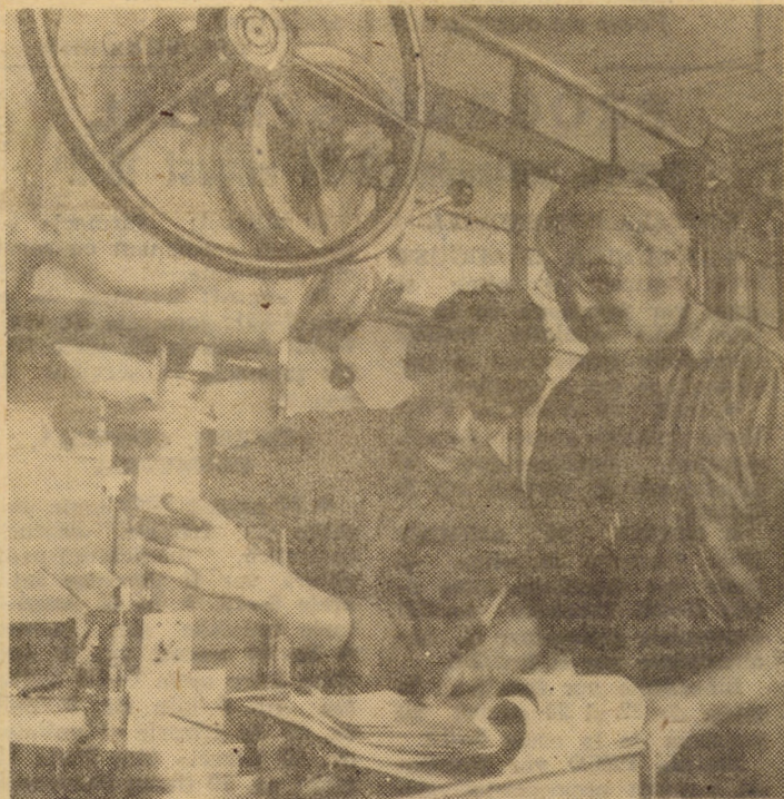
Mașină de găurit și frezat în secția scularie a întreprinderii mecanice Sibiu. Se prelucurează matrite de mare complexitate și precizie, necesare atelierelor de producție
