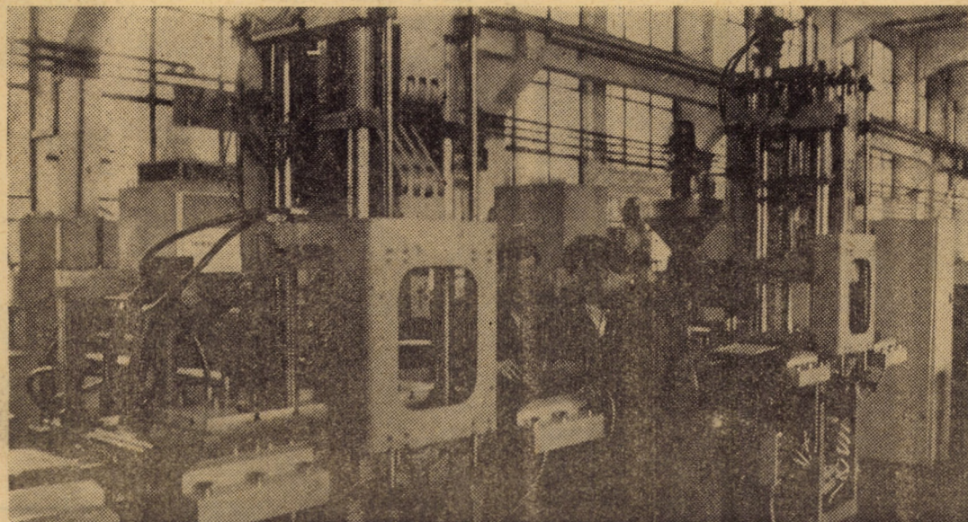
În secția sculărie a întreprinderii mecanice Sibiu se află în probe tehnologice un grup de mașini de injectat mase plastice cu închidere verticală și comandă program. Cu ajutorul acestor utilaje moderne se pot injecta mase plastice peste armături metalice. Prima mașină de acest gen va fi livrată beneficiarilor din industria electrotehnică în aceste zile
