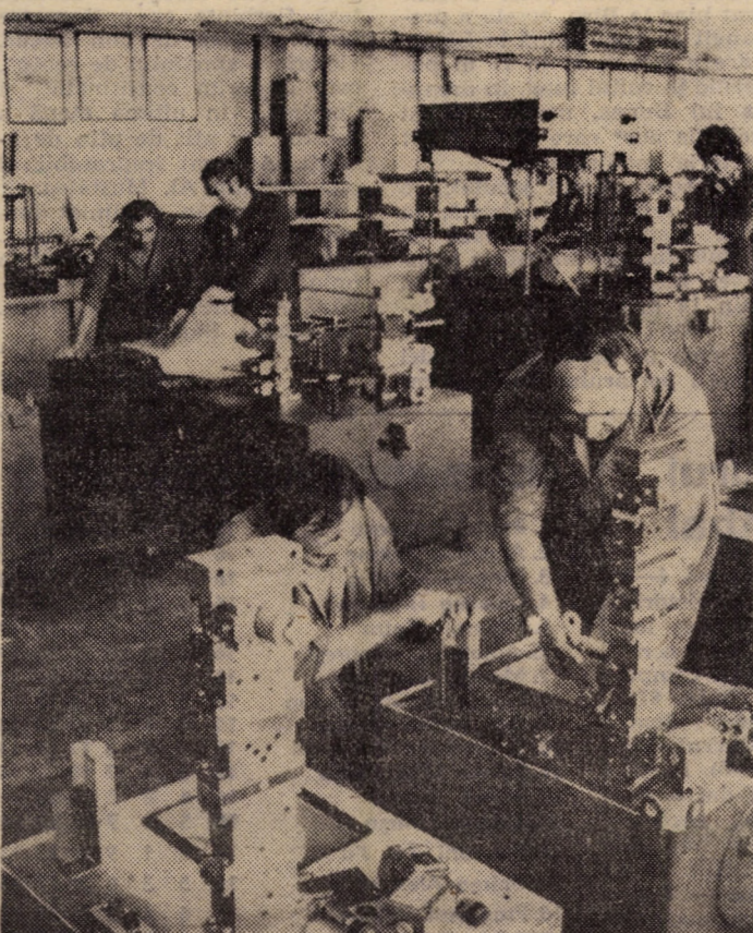
Montarea panourilor hidraulice la Fabrica de elemente hidropneumatice din Sibiu, componente necesare agregatelor și mașinilor unelte din industria constructoare de mașini Foto: Fred NUSS
