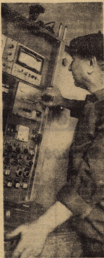
Verificarea parametrilor funcționali ai mașinilor de găurit la standul de probă din secția unelte pneumatice a întreprinderii „Independența” Sibiu.
