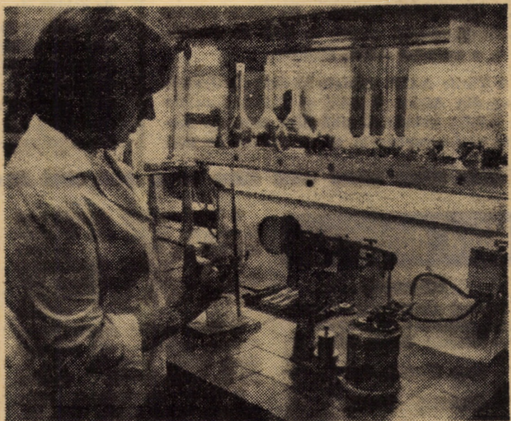
Determinarea indicelui de fluiditate la mase plastice în laboratorul de analize al întreprinderii „Flamura roșie” Sibiu. Foto: Fr. NUSS
