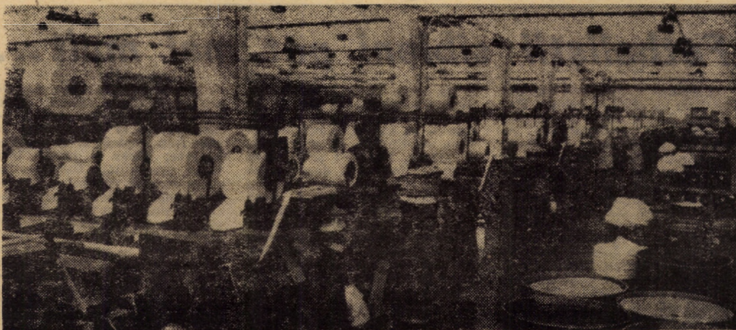
Întreprinderea „Firul roșu” Tălmăciu. Realizarea semitortului pentru mașinile de filat cu inele în secția filatură cu ajutorul mașinilor Flyer. Foto: Fred NUSS
