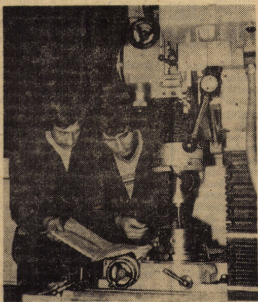
Întreprinderea mecanică Mediaș: muncitorul Nicolae Suciu și maistrul Aurel Ilea verifică exactitatea pieselor executate pe mașina de rectificat prin coordonate. Foto: Fred NUSS
