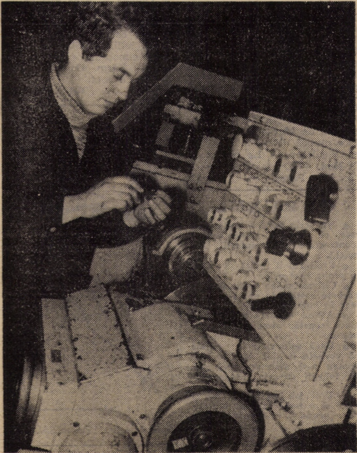
O bună parte din organele de asamblare pentru autoturismele „Dacia” și „Oltcit” se execută la întreprinderea mecanică din Mediaș pe strunurile automate cu comandă numerică. În imagine: utecistul Onichie Moldovan deservind un astfel de utilaj
