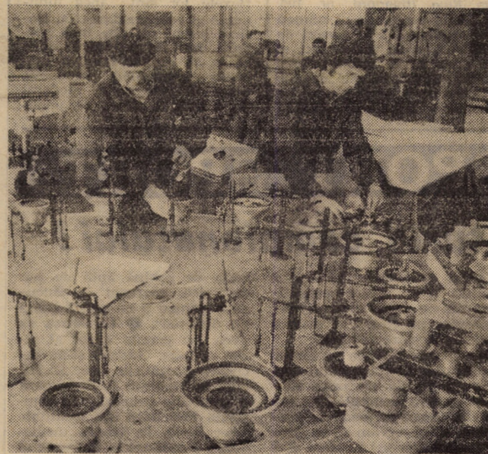
Lăcătușii Ioan Suciu și Otto Höhr fac ultimele probe la un utilaj ce urmează a fi expedit întreprinderii de porțelan din Alba Iulia
