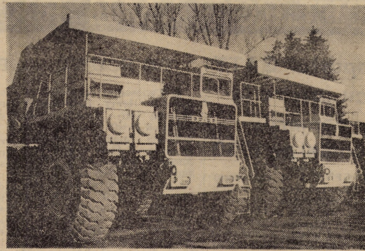
Din seria „giganților” construiți la Întreprinderea mecanică Mirșa: autobasculare de 110 tone Foto: Fred NUSS
