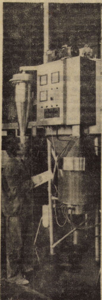
Instalație pentru fabricarea pudrelor de pigmenți la întreprinderea „Email roșu” Mediaș
