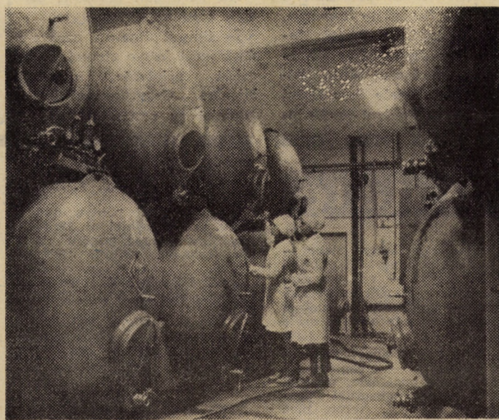
Instalații complexe de fabricarea berii în atelierele de producție ale Liceului industrial nr. 5 din Sibiu Foto: Fred NUSS
