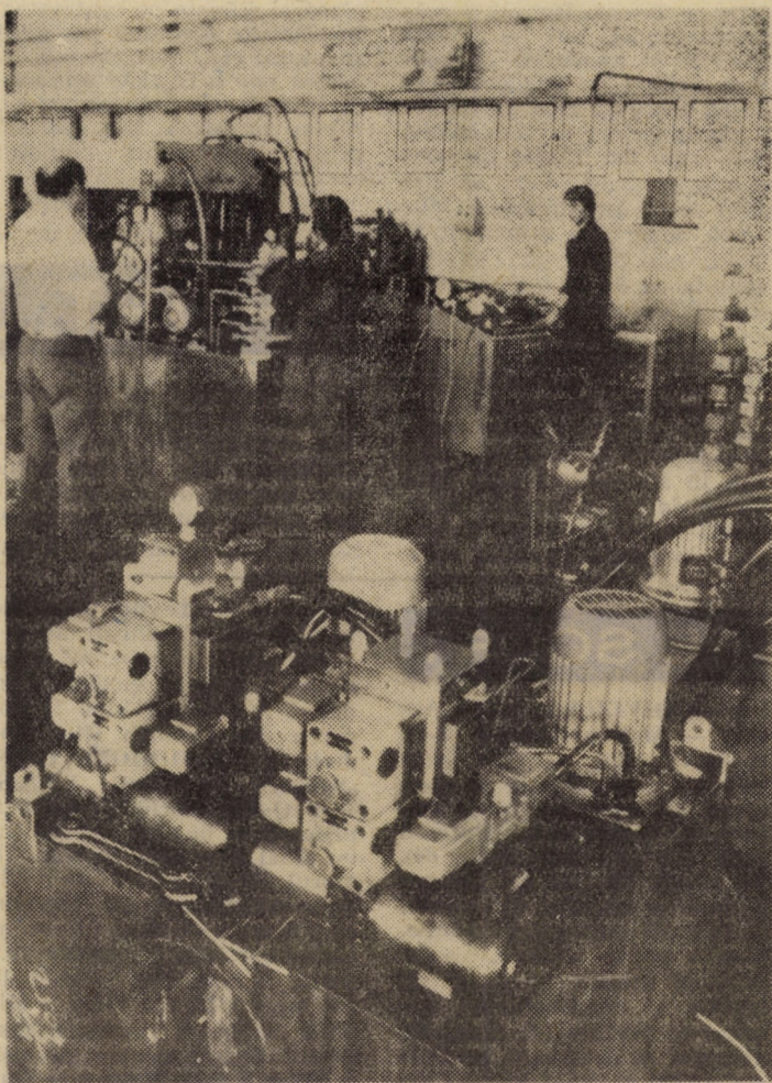
Lucrări de montaj în atelierul panouri hidraulice necesare mașinilor unelte și agregate la Fabrica de elemente hidropneumatice din Sibiu Foto: Fred NUSS
