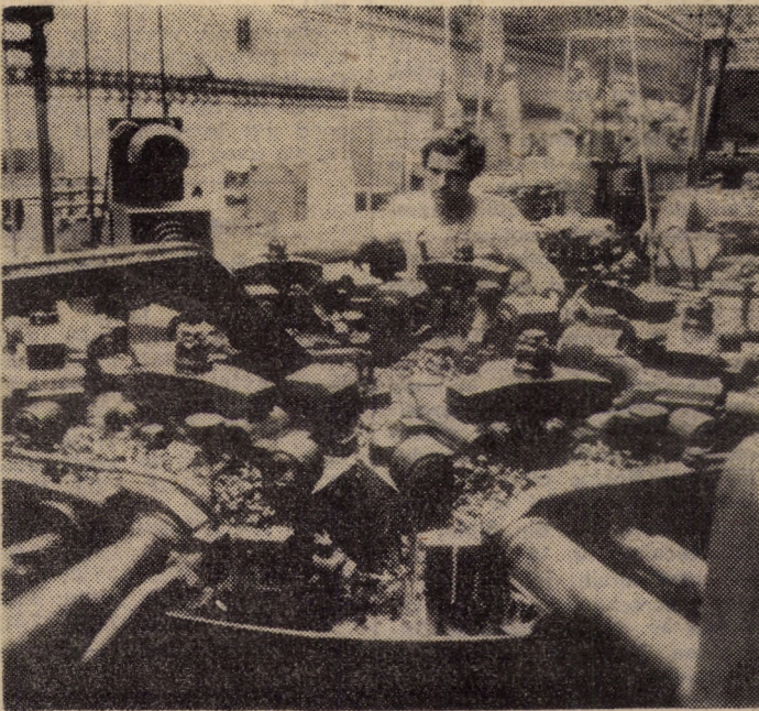
Imagine dintr-un important sector al I.P.A. Sibiu — prelucrări mecanice de înaltă precizie. Foto: Fred NUSS
