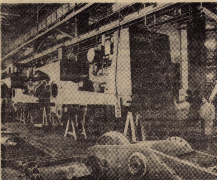
Linia de montaj a autobasculantelor de mare tonaj la I. M. Mirșea. Foto: Fred NUSS
