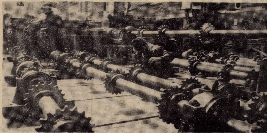
Asamblarea componentelor pentru utilaje grele în secția mecanică III a întreprinderii „Independența” din Sibiu. Foto: Fred NUSS
