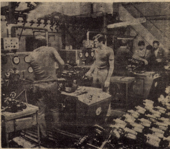
I.P.A. Sibiu. Standuri de probă finală a servodirecției hidraulice pentru autocamioane și autobuze. Foto: Fred NUSS
