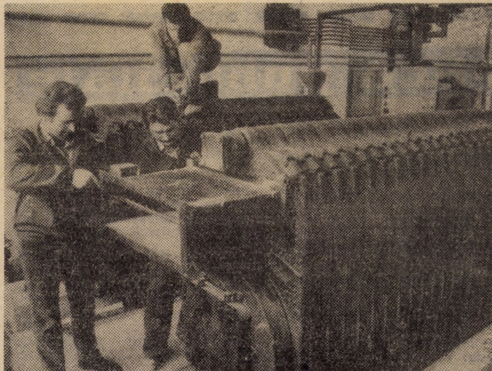
Specialiștii sectorului de exploatare al E.P.C.F.L. Sibiu acționează susținut pentru realizarea în termenele stabilite a reparației centralelor termice de cartier. În aceste zile a început montarea la centrala termică nr. 1 din Hipodrom (vezi foto) a două agregate „Gaz - 900“ pentru cazane, care obțin un randament termic superior vechilor instalații. Pînă la începutul sezonului rece se vor monta încă 4 asemenea agregate pentru cazane la centrala termică din cartierul Tîglari și cîte două la C.T. Ștrand (vechi) și C.T. 5 Hipodrom
