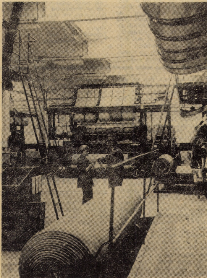
Aspect din secția covor plușat a întreprinderii „Textila” Cîsnădie
