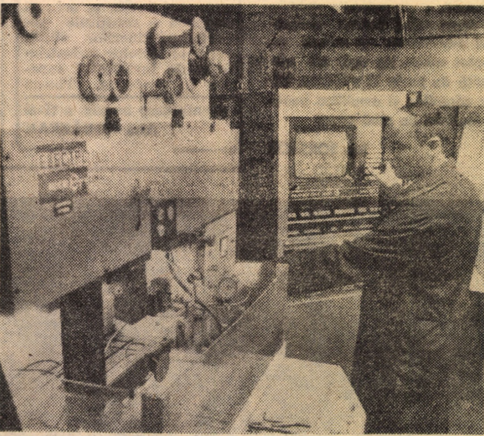
În secția prototipuri a întreprinderii „Flamura roșie” Sibiu, o mașină de prelucrat prin electroeroziune cu fir de tip „ELEROFIL 10”, produsă de „ELECTROTIMIȘ” Timișoara, asigură execuția unor matrice cu profile de un înalt grad de complexitate,
