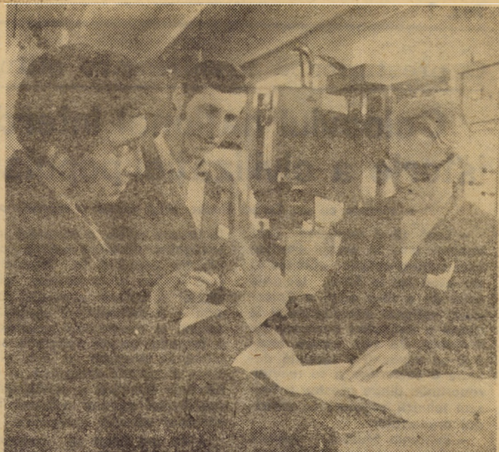
Prin folosirea mașinilor de prelucrare prin electroeroziune în secția sculărie a întreprinderii „Flamura roșie” Sibiu se obține întreaga gamă de S.D.V.-uri cu profile complexe în oțeluri tratate termic și carburi metalice, necesare procesului de producție. În fotografie: comunistul Vasile Chinceș, maistrul de schimb (dreapta), alături de operatorii Hermann Burtesch și Karol Pfaff analizând modul de prelucrare a unor noi matrițe Foto: Fred NUSS
