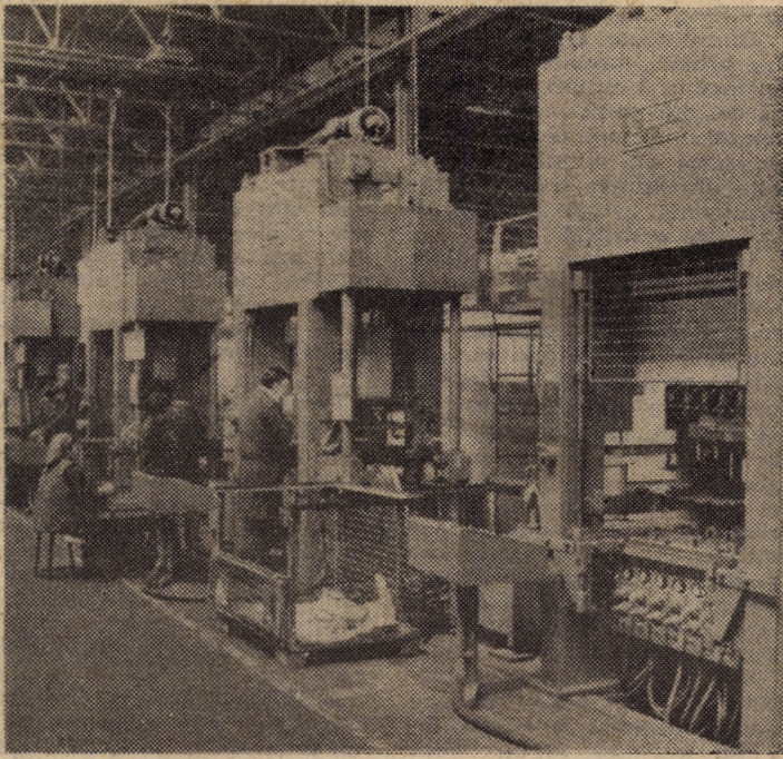
Linia de prese cu transfer în secția ambutasat a întreprinderii „E-mailul roșu”, Medias. Foto: Fred NUSS
