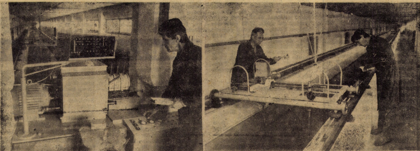
Institutul de meteorologie și hidrologie, colectivul de aparatură Sibiu dispune, printre alte instalații, și de un canal hidrostatic cu o lungime de 68 metri cu ajutorul căruia se efectuează lucrări de cercetare și testare pentru moriștile hidrometrice, folosite în calcularea vitezei de scurgere a apelor. Înregistrarea parametrilor se face atât mecanic cit și electronic. În cele două imagini ing. Octavian Rădulescu și tehnicianul principal Orest Ivașcu în timpul unei testări la canalul hidrostatic
