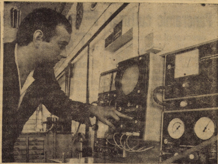
La noua stație service A.C.R. din Sibiu, testarea și reglarea motoarelor autoturismelor se efectuează cu ajutorul unei aparaturi de înaltă tehnicitate. În fotografie: mecanicul Eugen Streza lucrînd la testerul electronic Foto: Fred NUSS
