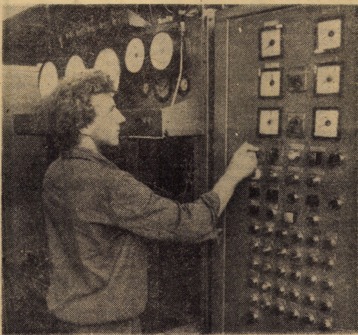
Întreprinderea de elemente hidropneumatice Sibiu. La unul din standurile de probă pentru verificarea supapelor și distribuitorilor hidraulice lucrează și comunistul Dan Roman, absolvent al Liceului industrial. În cursul celor 3 ani de când s-a încadrat, dînd dovadă de pricepere și hărnicie, el s-a alăturat tinerilor cu bune rezultate în producție. Foto: Fred NUSS
